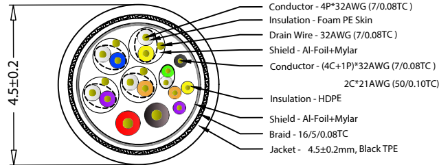
SEC:A--A'
